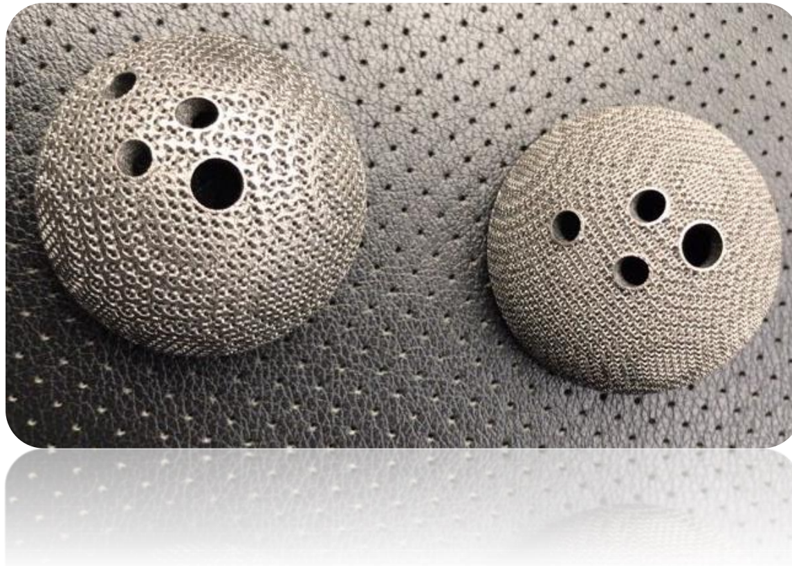
3D打印定制化钛合金髋臼假体
